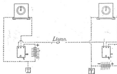
Fig. 184. — Schema du montage dans le cas d'un transmetteur et d'un récepteur à chaque poste.
